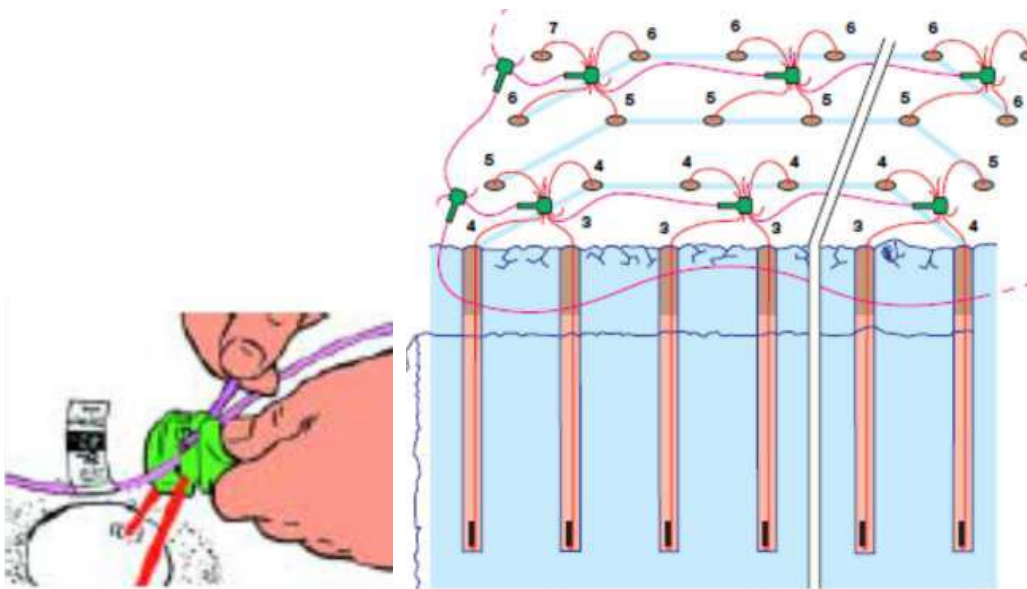
Слика 14. Поврзување на нонел цевки Слика 15. поврзување на минска серија со помошна конектор (спојка)
