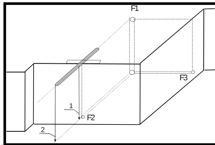
Слика 21. Одредување на правец на хоризонтална дупчотина
