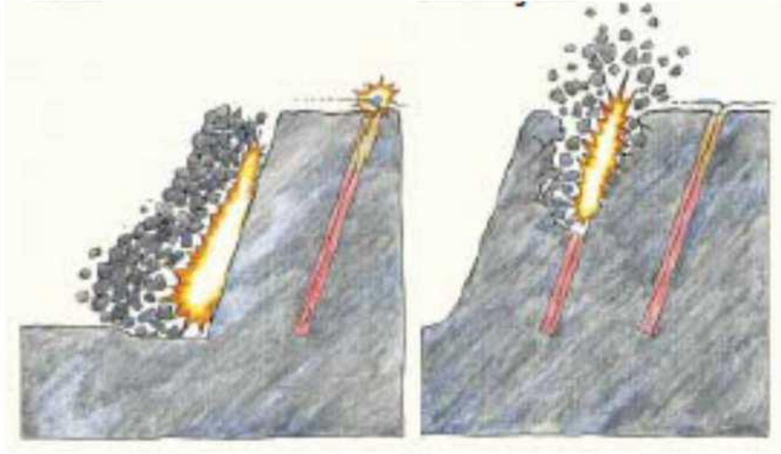
Слика 13. Минарање со Нонел систем и минарање со детонаторски фитил
