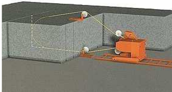
Слика 24. Пилење на вертикални резови
