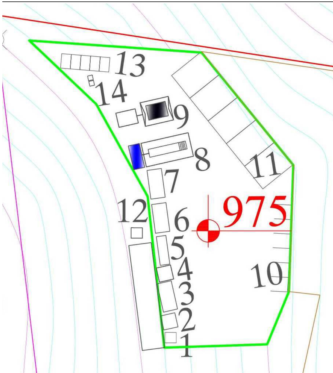
Слика 4. Рудничко градежни објекти
