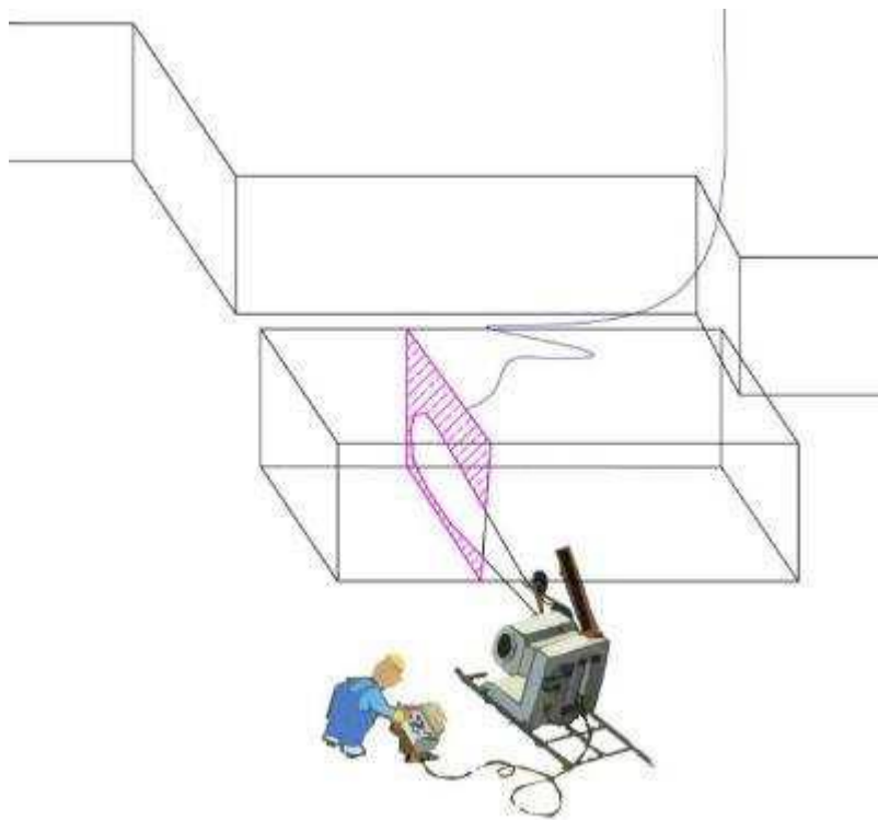
Слика 32. Плацно сечење со дијамантска жична пила TL 920
