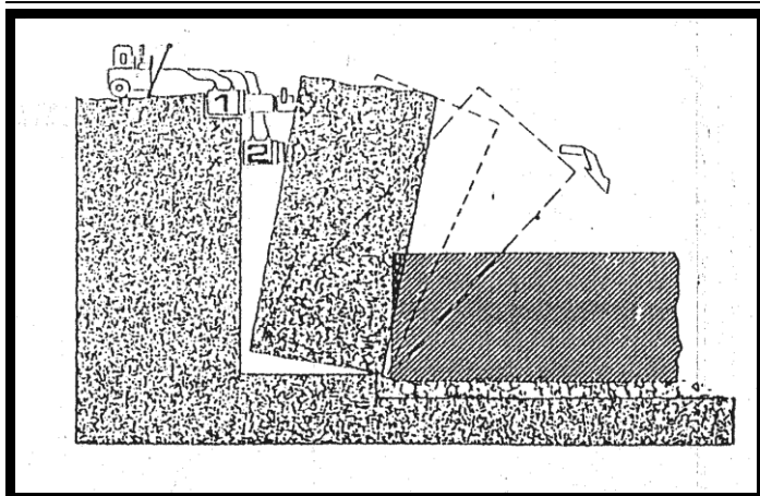
Слика 27. Соборување со хидраулични соборувачи
