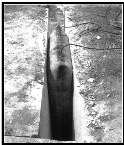
Слика 28: Соборување на ламела со воздушна перница
