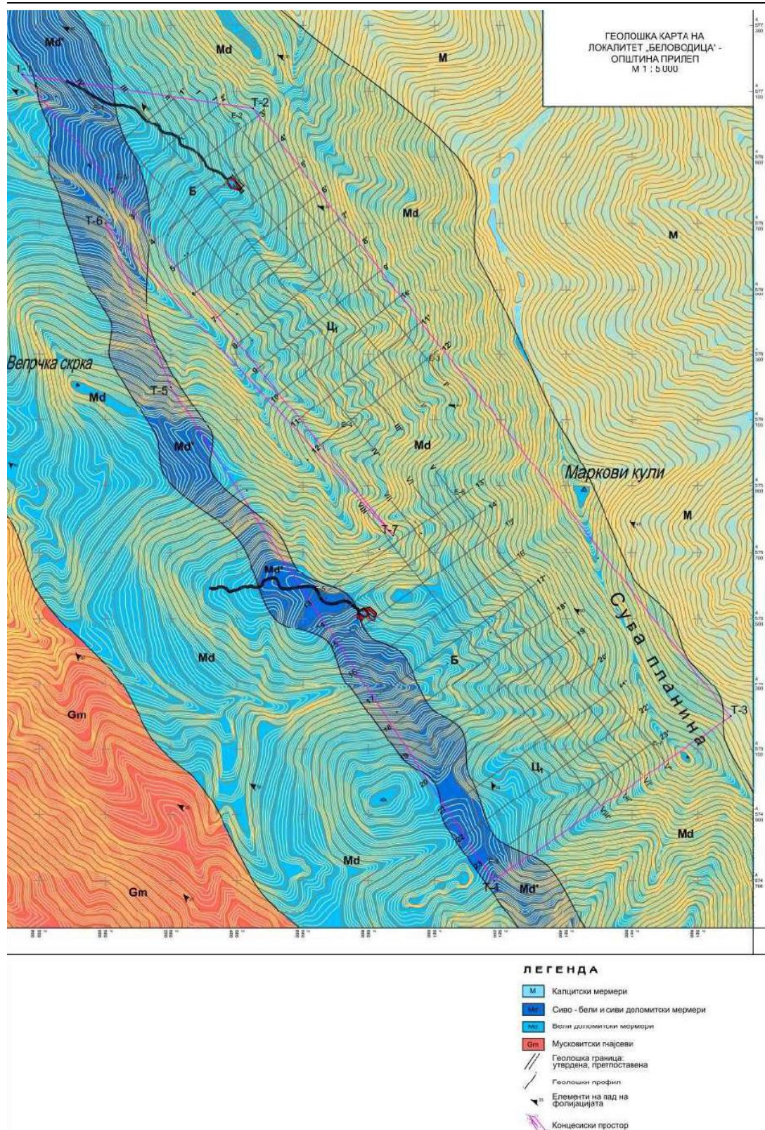
Слика 11. Геолошка карта на локалитетот Беловодица
