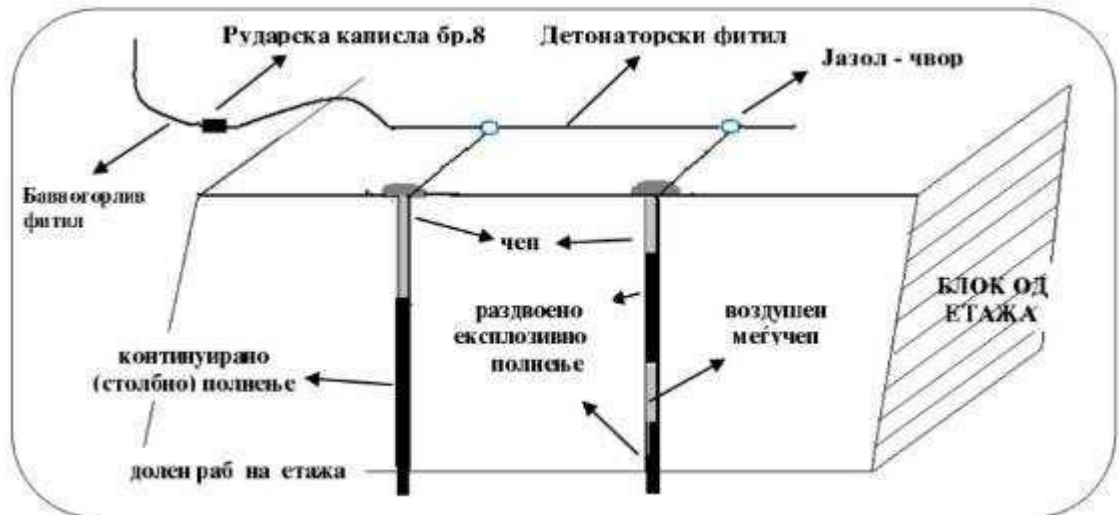
Слика 12. Шематски приказ на минско поле
