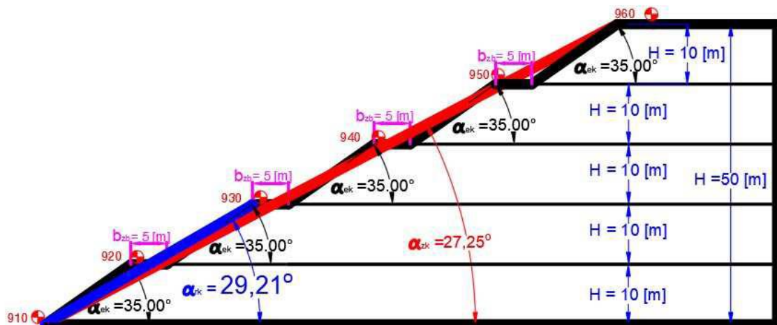
Слика 36. Профил на одлагалиштето во површинскиот коп “Беловодица”
