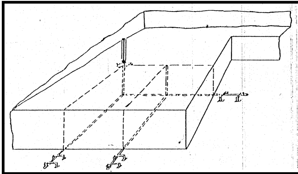
Слика 22. Дупчење на дупнатини за дијамантска жица
